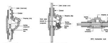
คอมปานด์ กันระเบิด
